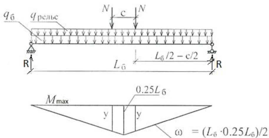
Рис. 3. – Схема мостового крана к проверочному расчету пролетной балки.
