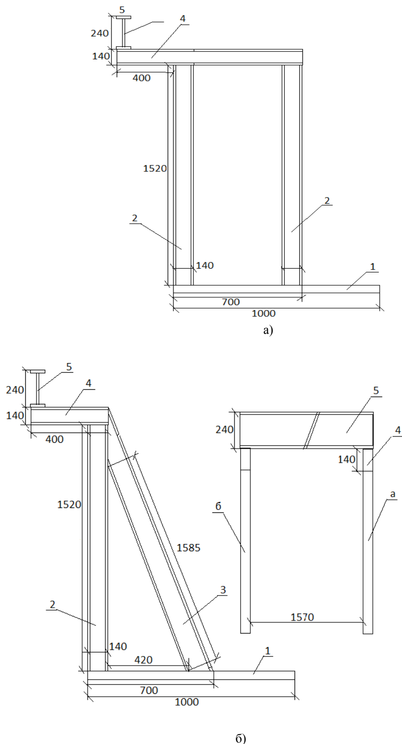
б) Рис. 2. – Обмерный чертеж узла крепления тали г/п 2 т. зав. № xxxx 1 - опора; 2 - с тойка; 3 - подкос; 4 - консоль; 5 - двутавр, направляющая тали [Measuring drawing of the fastening unit of the hoist rope 2 tons No. xxxx 1 - support; 2 - rack; 3 - hinge; 4 - console; 5 - I-beam, guide rail]
